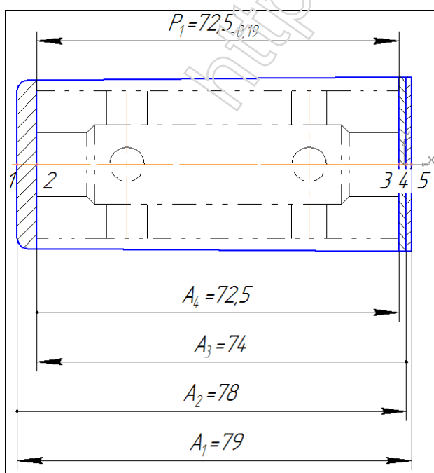
Рисунок 2 – Размерная схема
